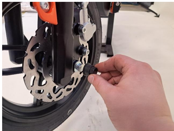
Ota tarvikepussista etuakselin päihin tulevat tulpat.
